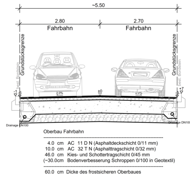
Regelquerschnitt Nord Station 0+070
