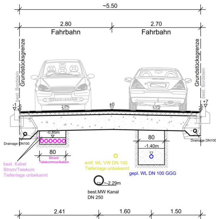
Regelquerschnitt Nord Station 0+070
